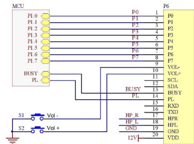
接続図：
