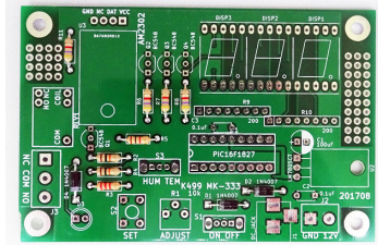
ダイオードのハンダ付け
