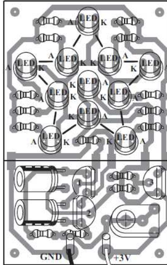
実体配線図
